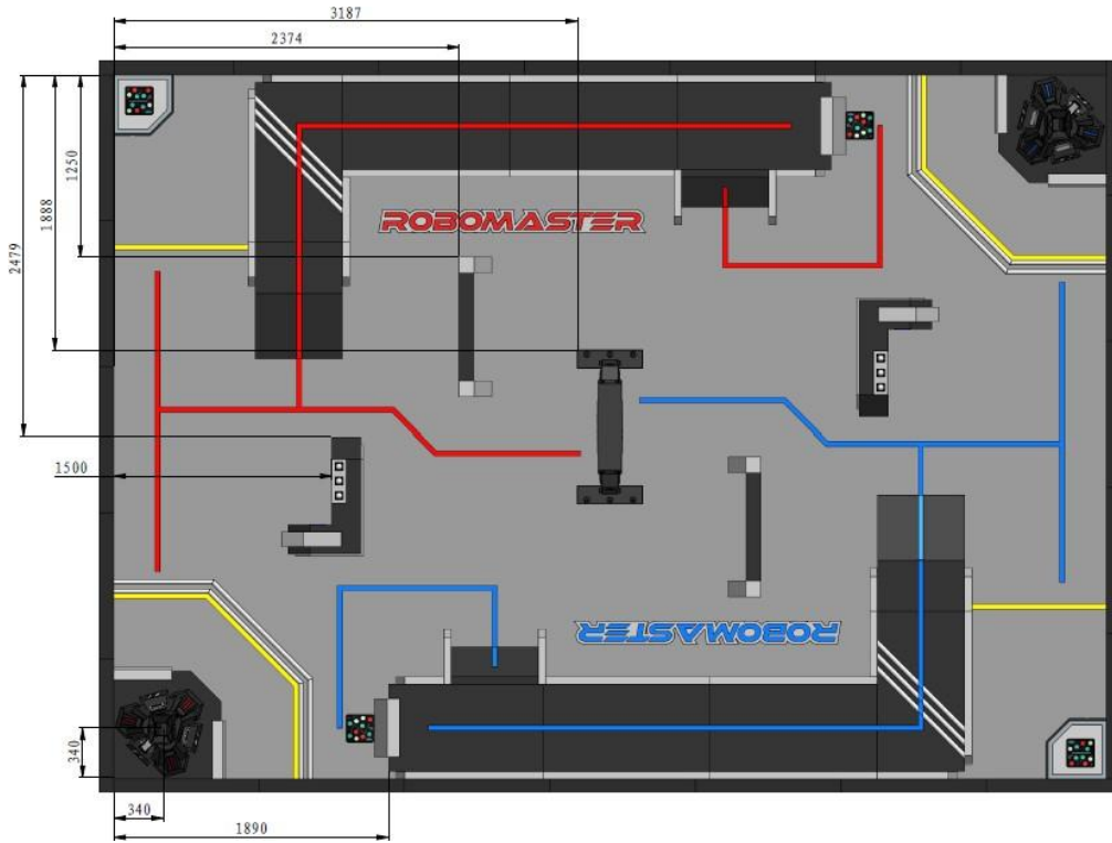
图 四-5 战场模块定位尺寸图
