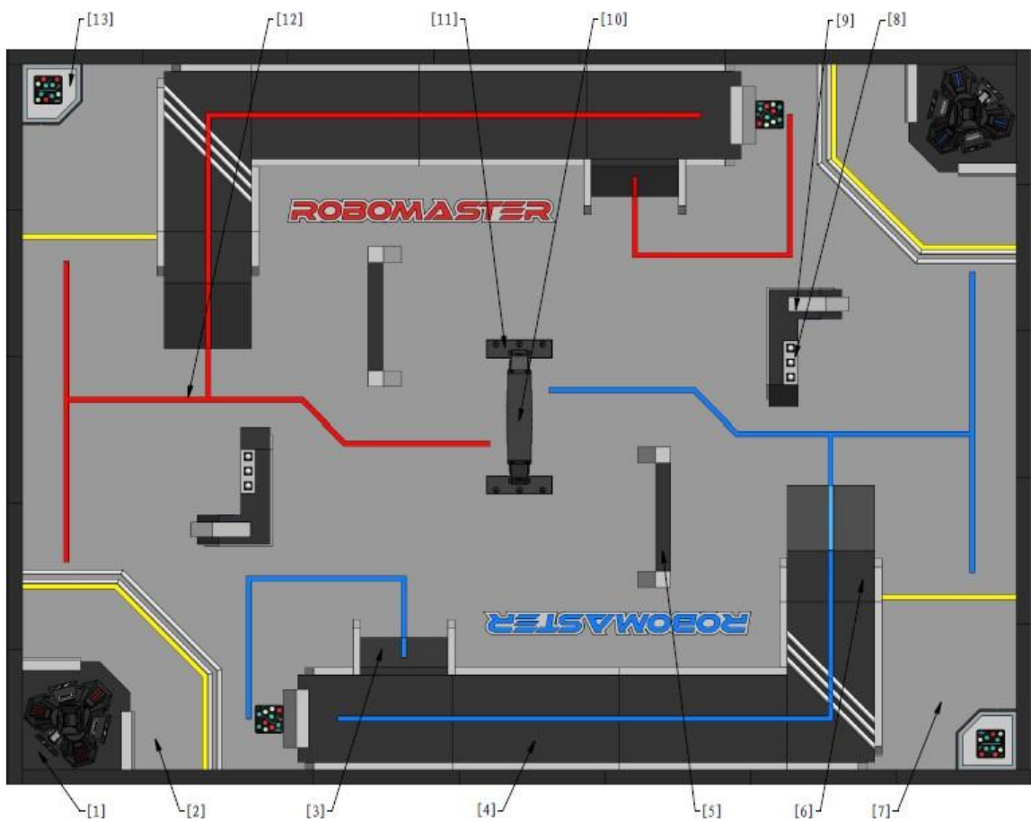
图 四-4 战场模块示意图
