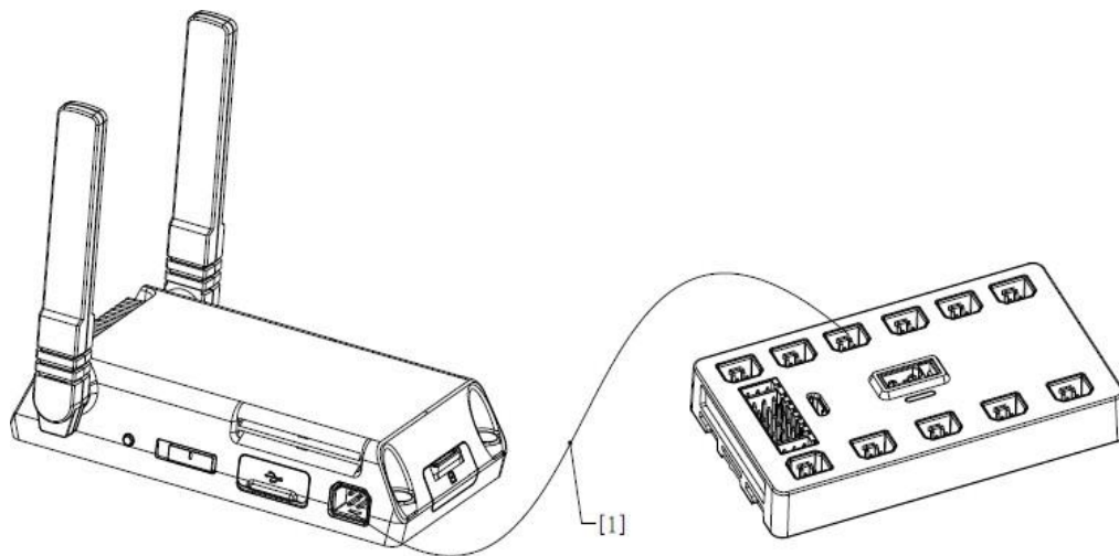
图 十-18 智能中控连线示意图
