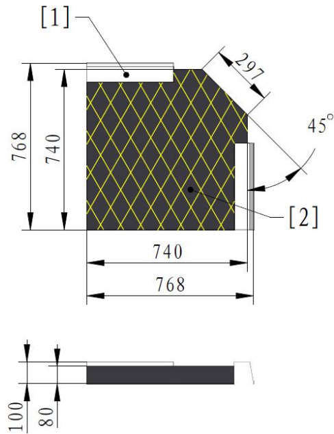
[1] 基地底座 [2] 基地禁区
