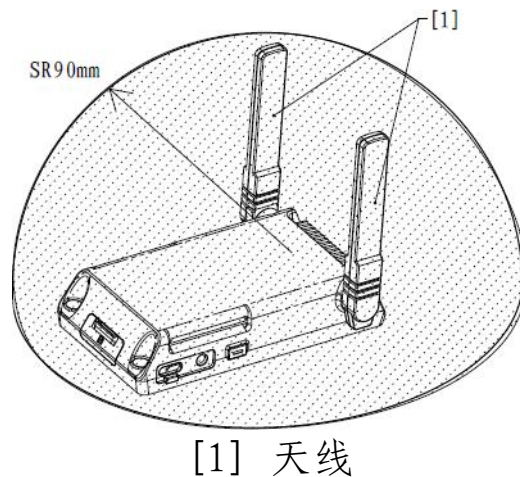
图 十-19 智能中控安装位置示意图
