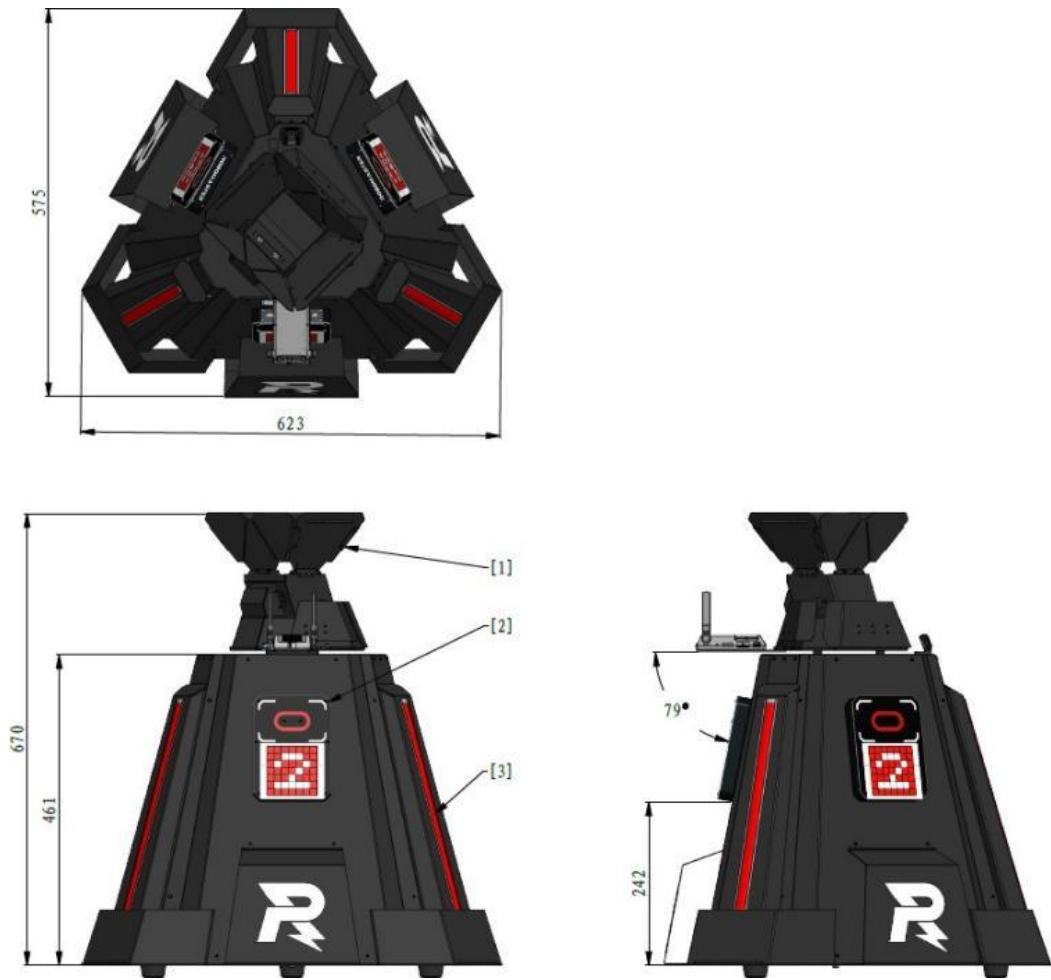
图 四-11 基地示意图
