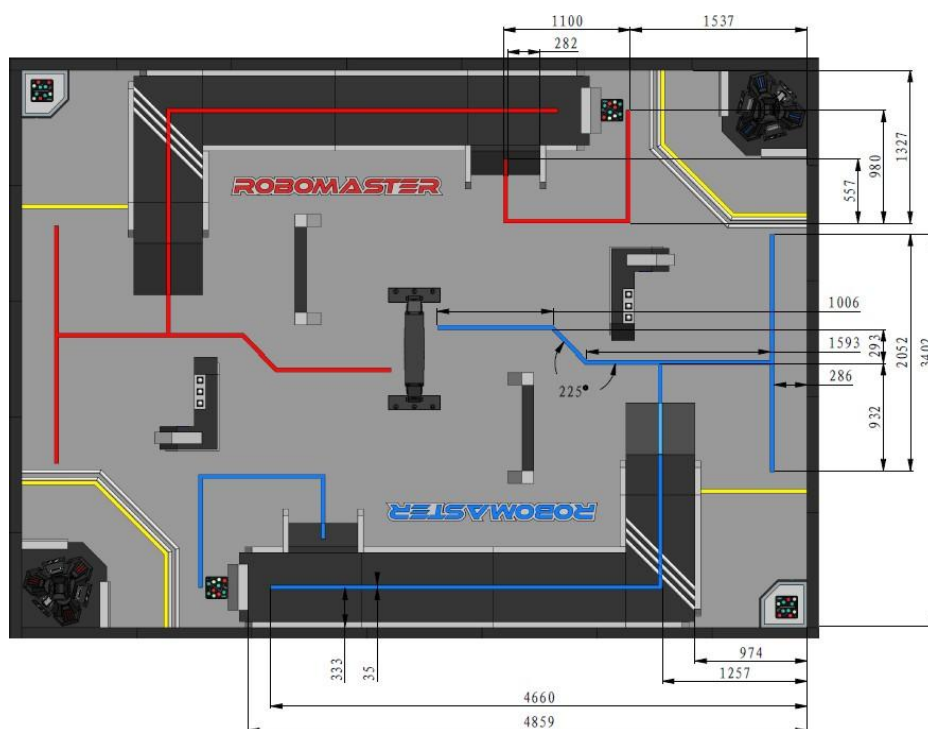
图 五-3 场地引导线
